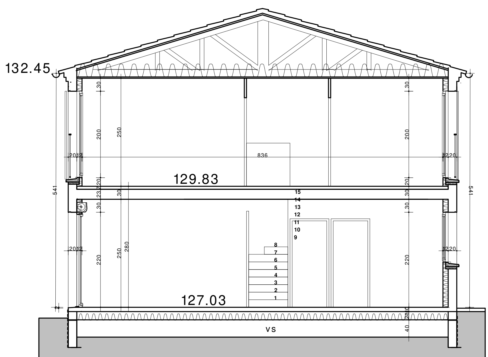
COUPE B-B
